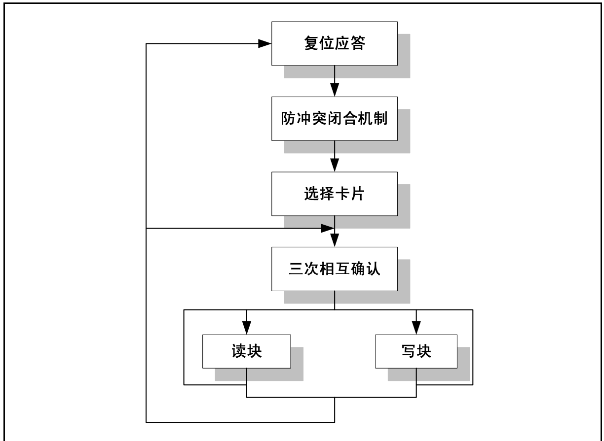
图 2-2 FM11RF32 操作流程
