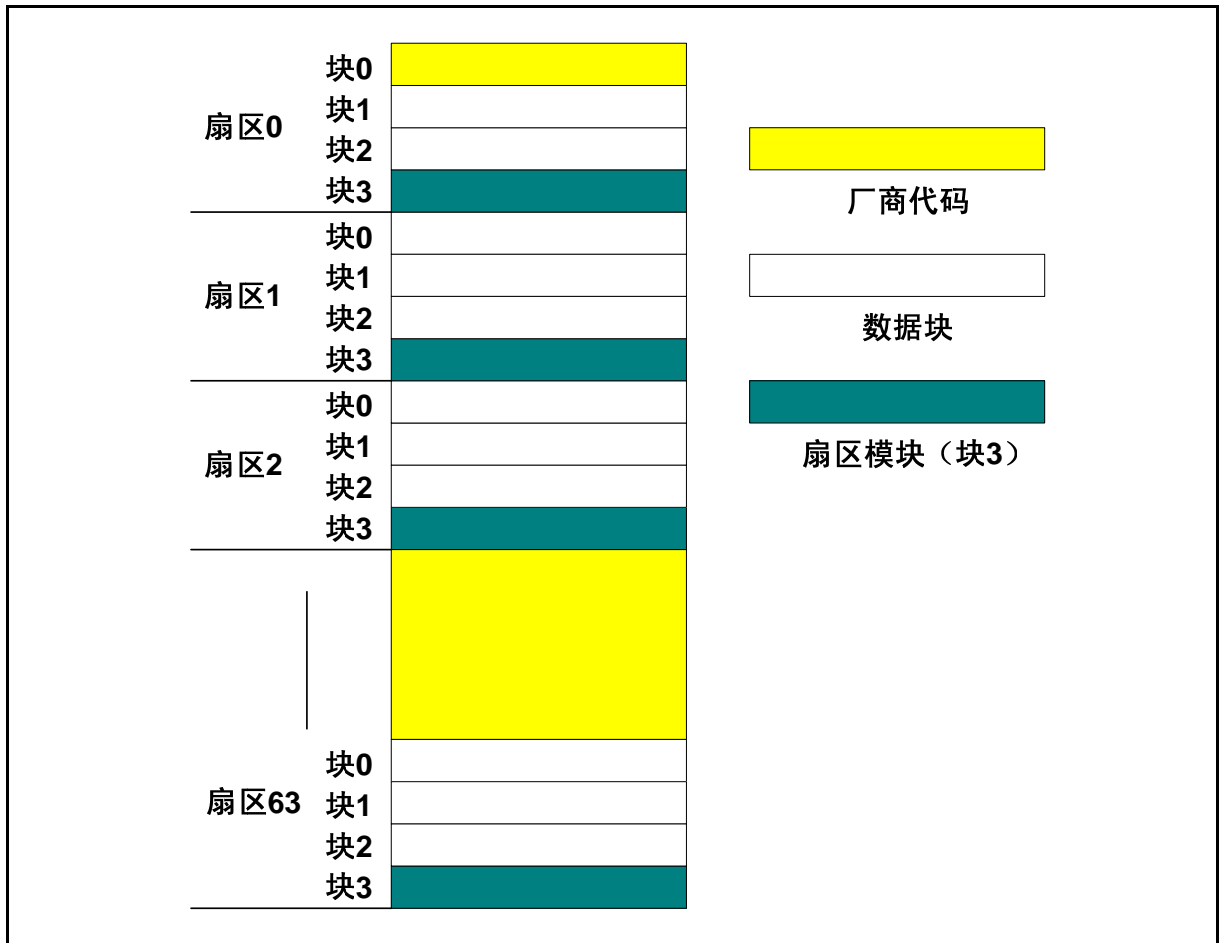
图 4-1 FM11RF32 存储器分区图
