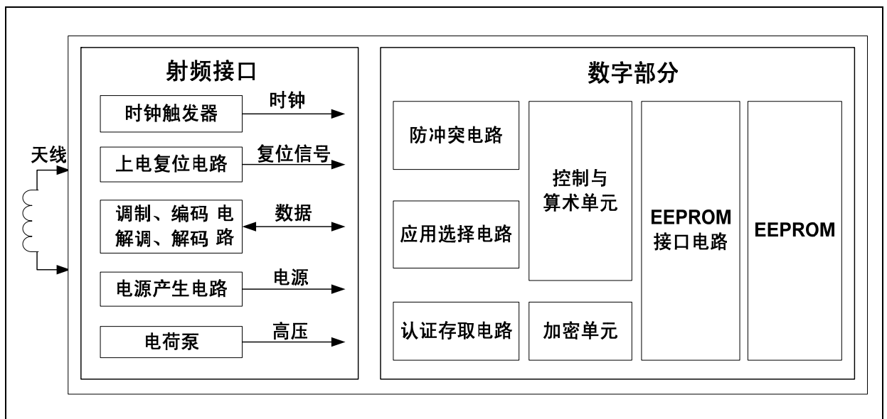
图 2-1 FM11RF32 功能框图
