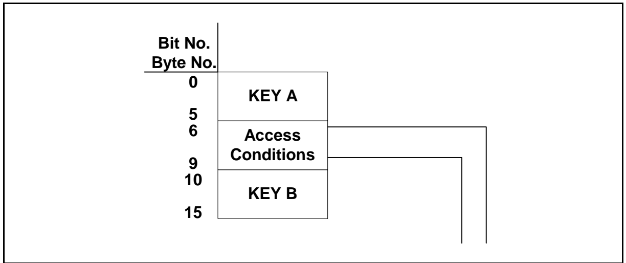
图 4-2 FM11RF32 存储器块 3 结构图
